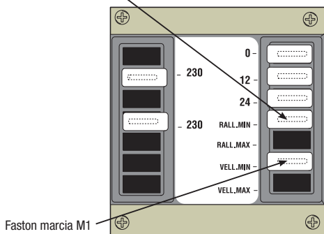
Faston rallentamento M1
